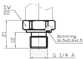
G ¼ A; DIN 3852; Form E
